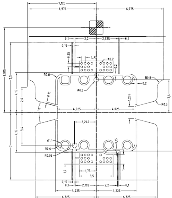
Рисунок 3. Обратная сторона чип-модуля
