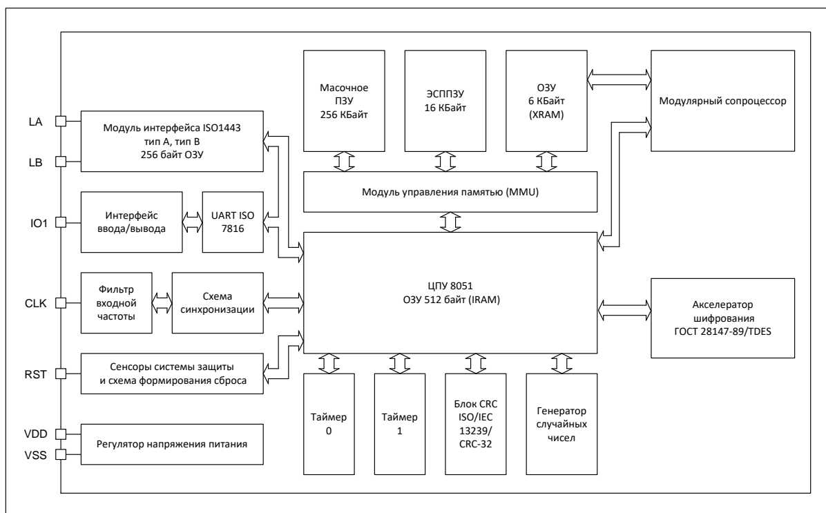
Рис. 1 Блок-схема микроконтроллера.
