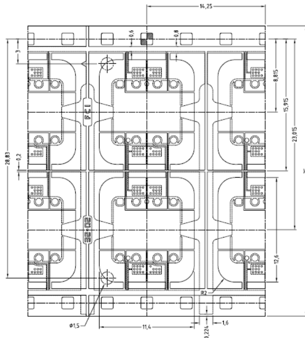
Рисунок 4. Расположение чип-модулей на ленте.
