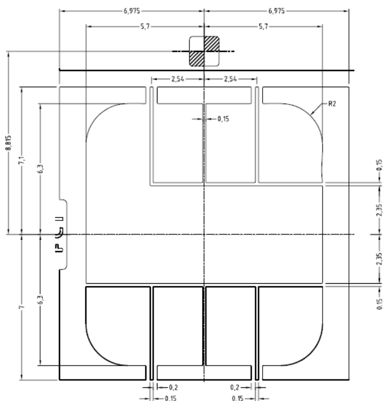
Рисунок 2. Лицевая сторона чип-модуля
