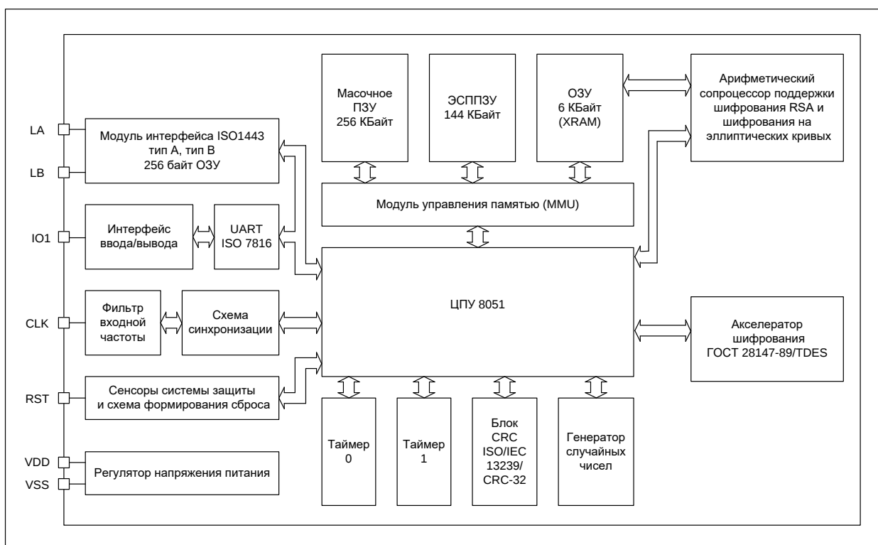
Рис. 1 Блок-схема микроконтроллера.
